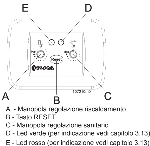
Figura 3-2 - Comando remoto
