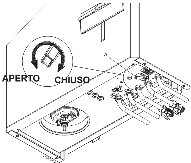
Figura 3-3 - Rubinetto di carico
