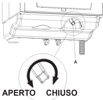
Figura 3 - Rubinetto di carico
