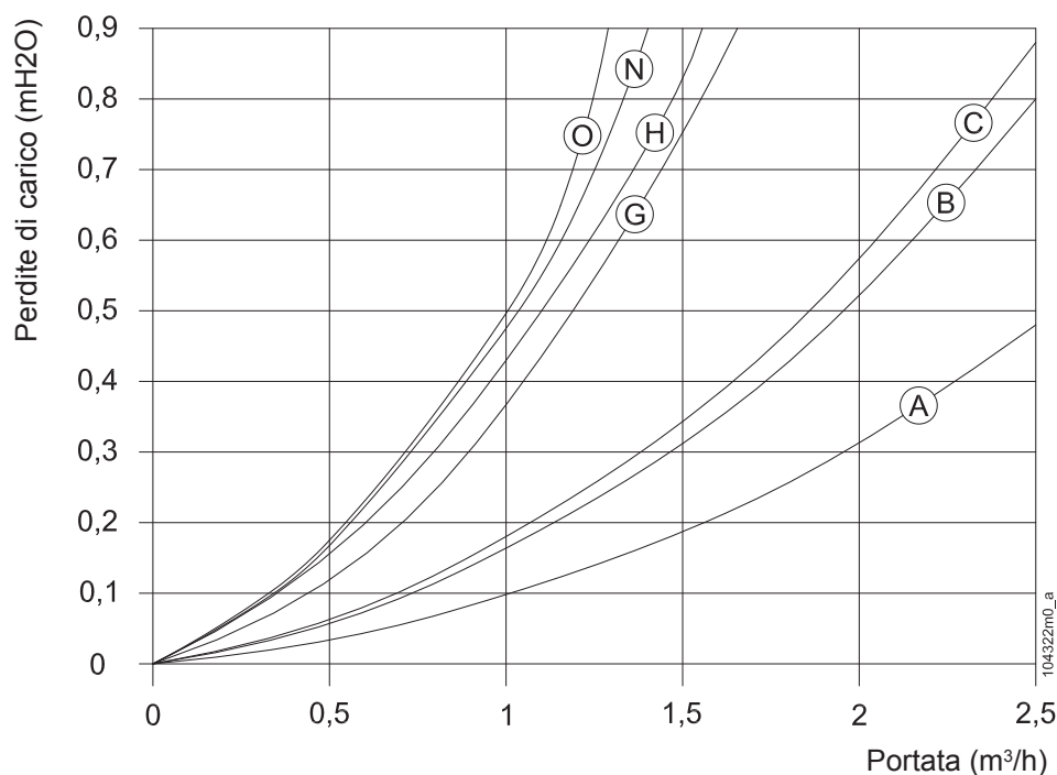
Figura 13 - Perdite di carico del serpentino inferiore
