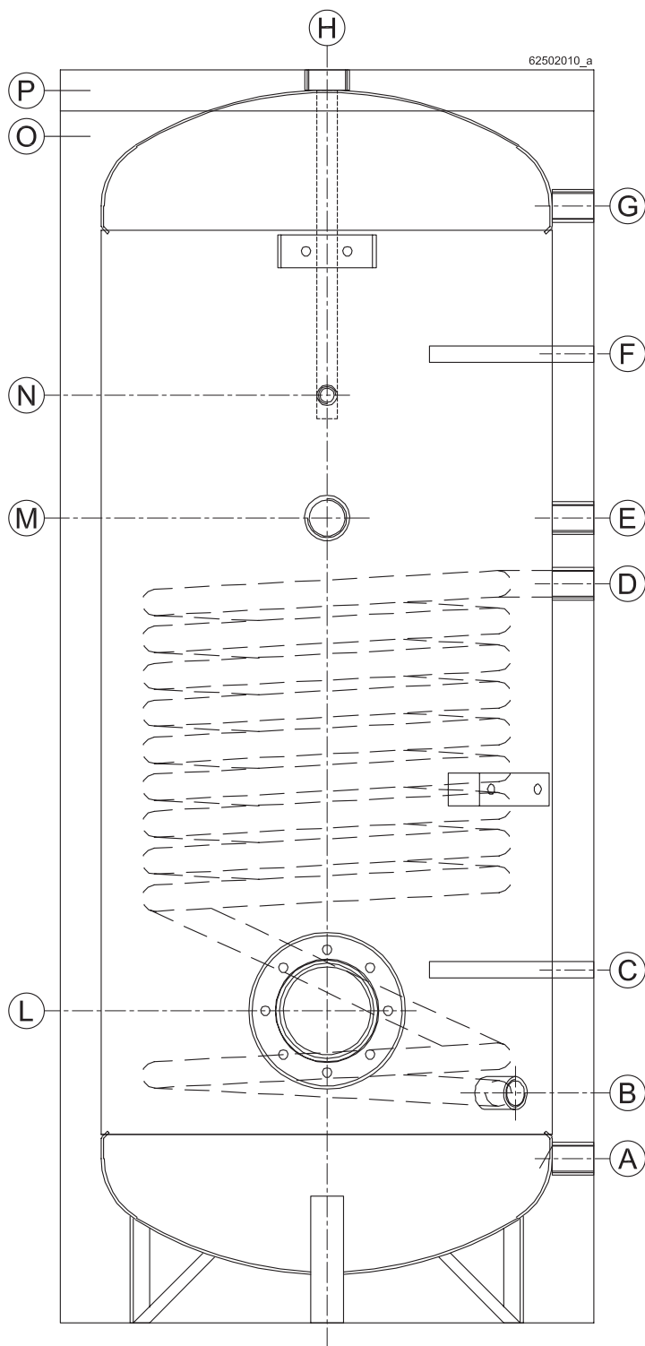
Figura 1 - Componenti principali bollitore BP/1
