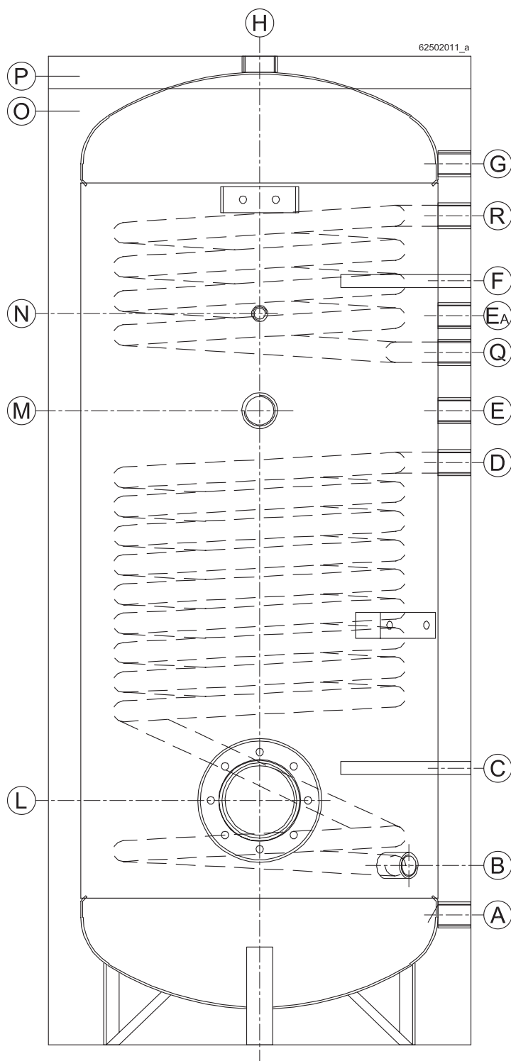
Figura 2 - Componenti principali bollitore BP/2
