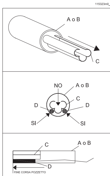
Figura 12 - Corretto posizionamento sonde
