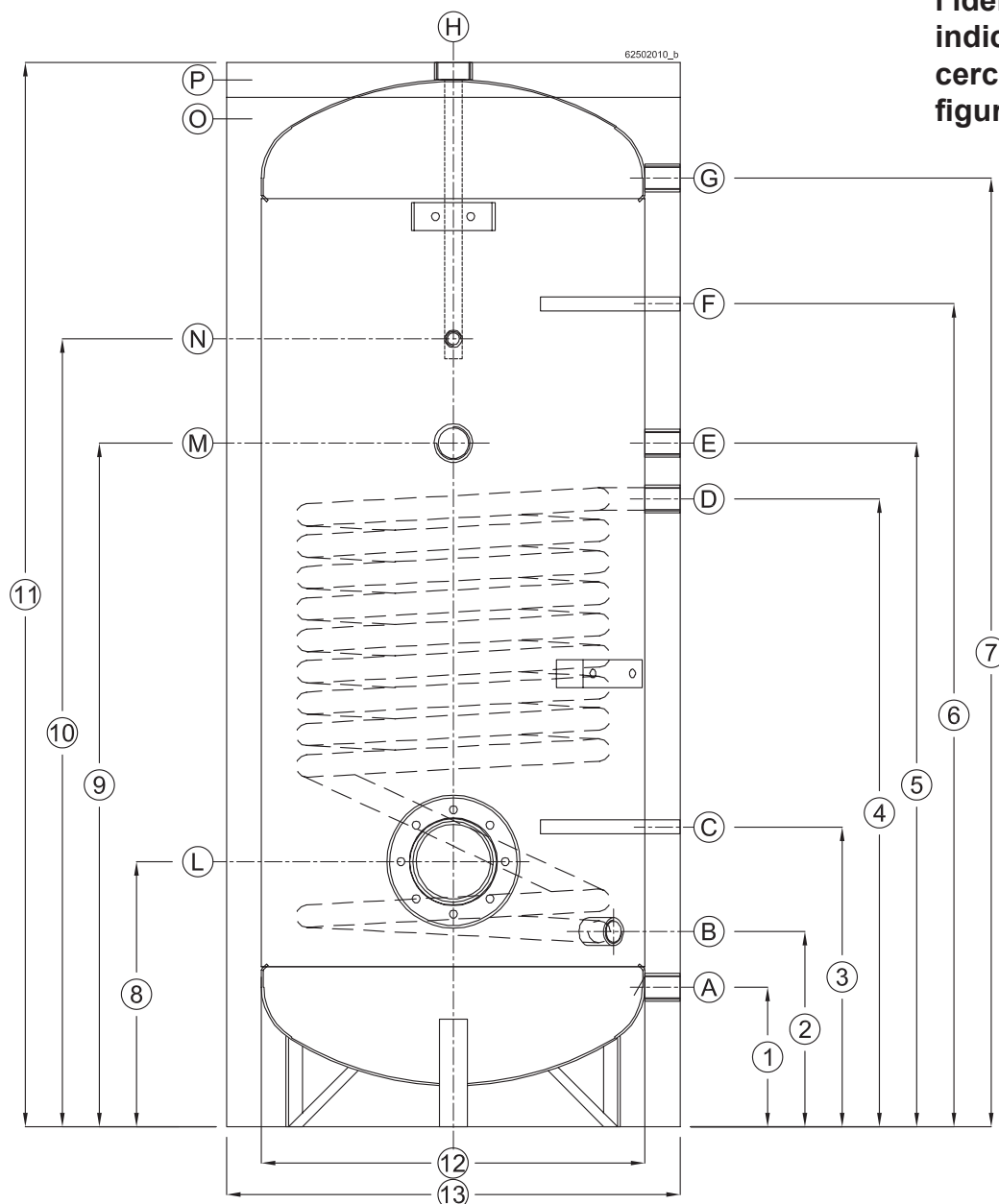
Figura 7 - Dimensionali bollitore BP/1 (riportate in mm al capitolo 4.3)
