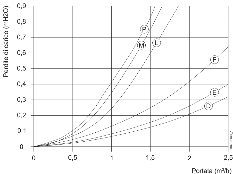
Figura 14 - Perdite di carico del serpentino superiore
